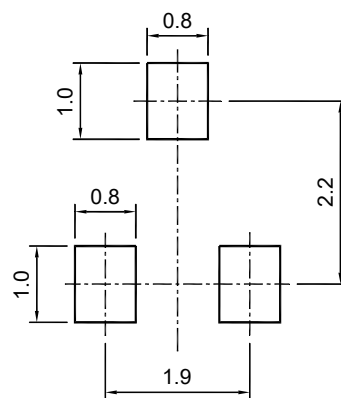
SOT-23
